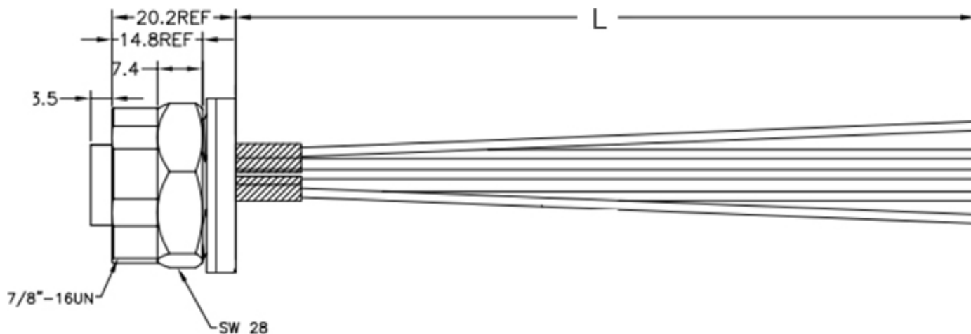
DIMENSIONS
