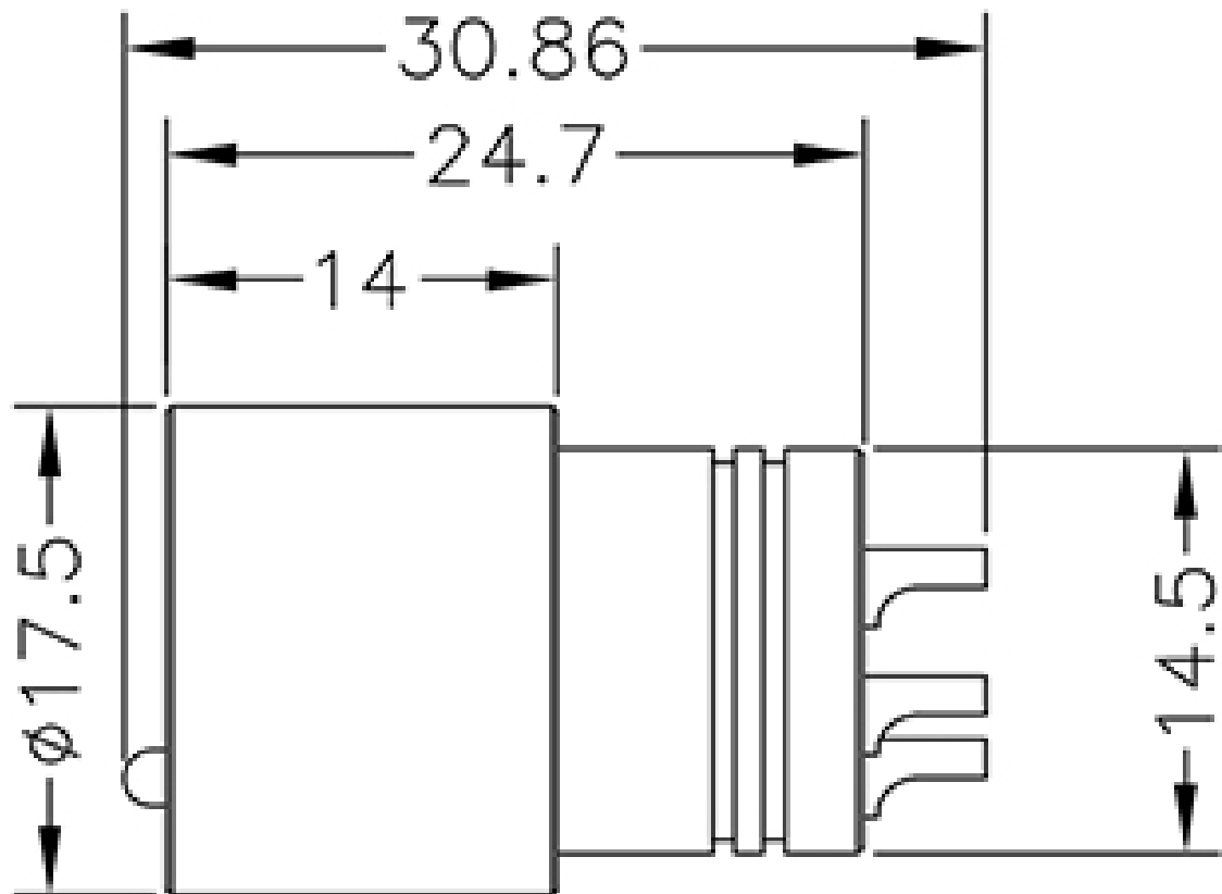
DIMENSIONS
