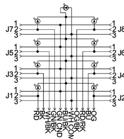
WIRING SCHEMATIC
