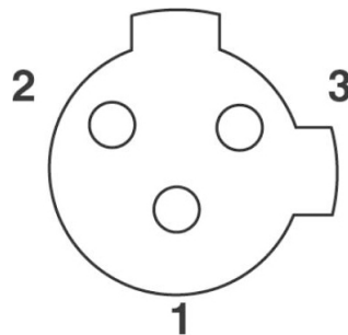
WIRING SCHEMATIC
