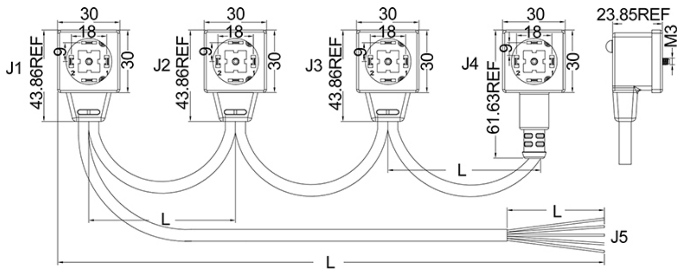
DIMENSIONS
