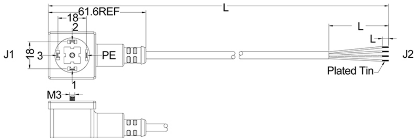
DIMENSIONS
